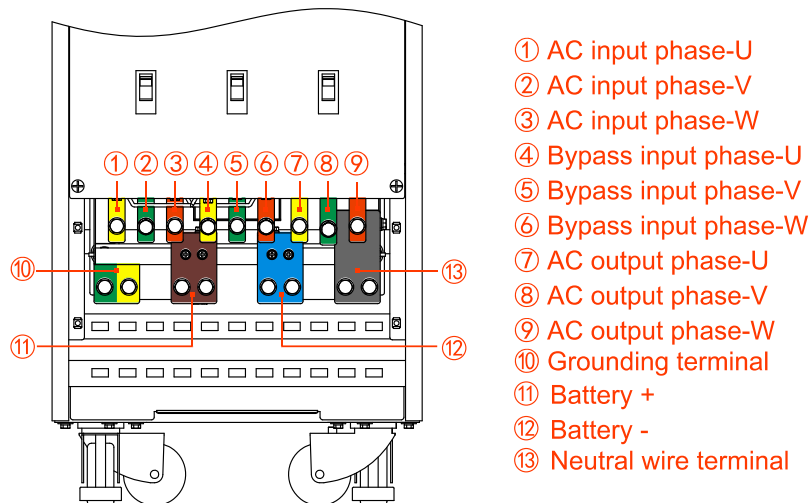
Рис 3.22 Схема подключения клемм для KR(/B)3380, KR(/B)33100, KR(/B)33120
