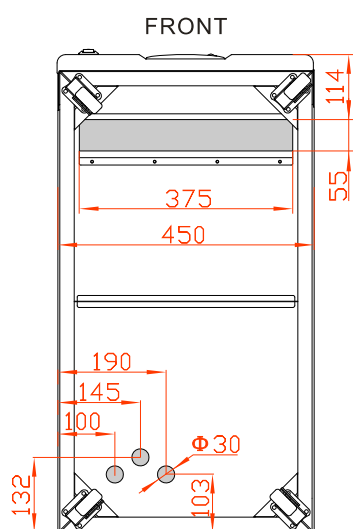
Рис 3.19 Схема нижних монтажных отверстий для KR(/B)3350, KR(/B)3360
