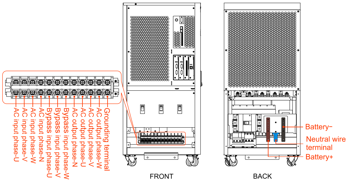
Рис 3.22 Схема подключения клемм для KR(/B)3350, KR(/B)3360
