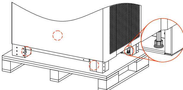
Рис 3.9 Позиция болтов
