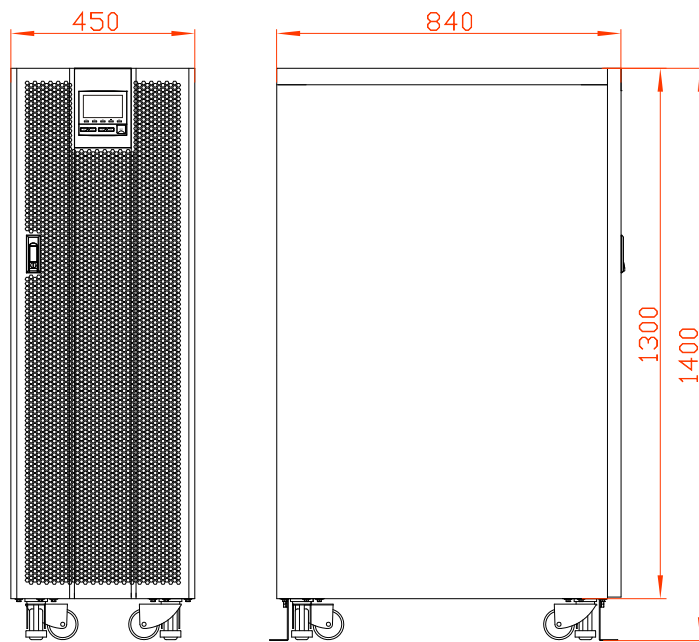
Рис 3.12 Размеры для KR(/B)3380, KR(/B)33100, KR(/B)33120
