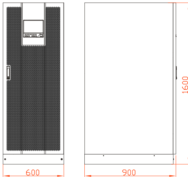
Рис 3.14 Размеры для KR(/B)33160, KR(/B)33200
