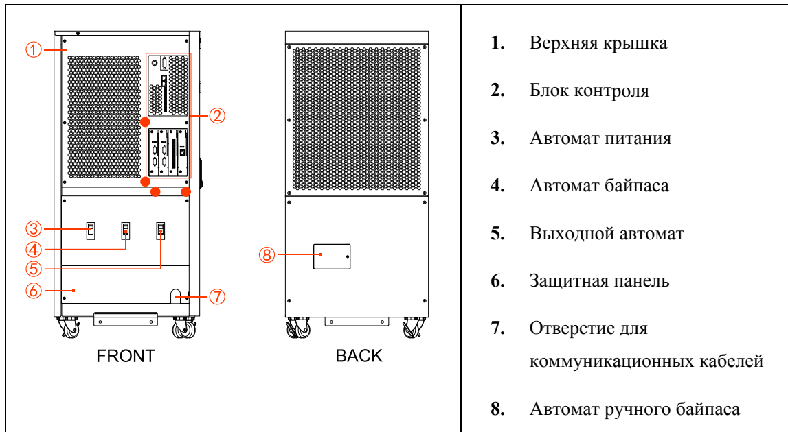
Рис 2.9 Структурная схема расположения для KR(/B)3350, KR(/B)3360
