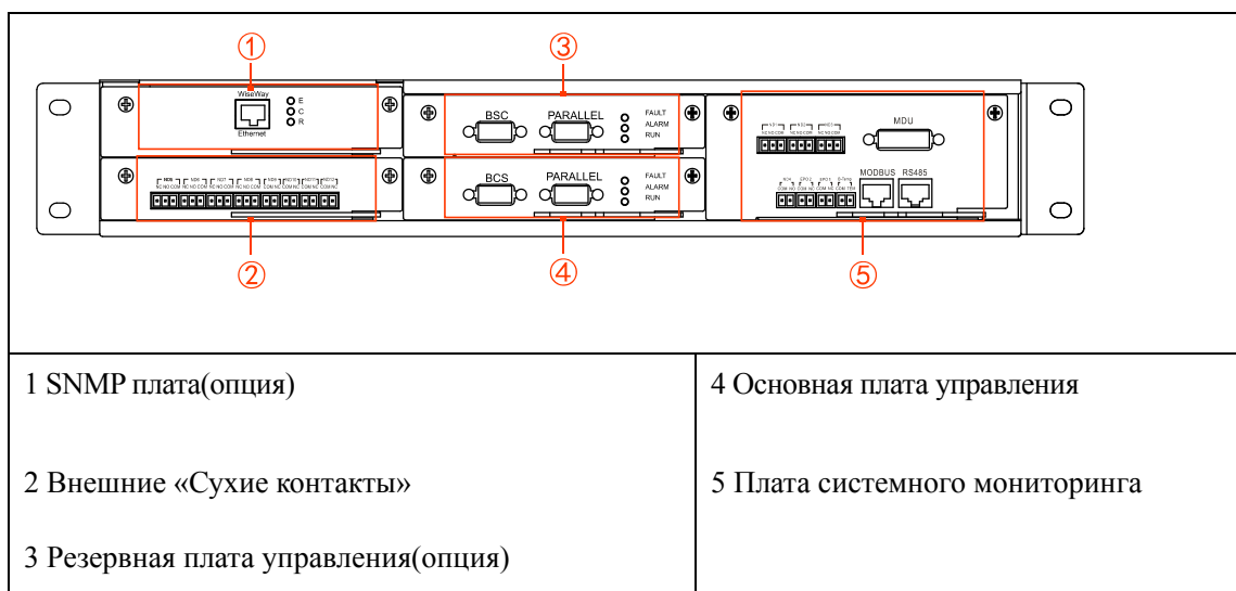
Рис 2.15 Блок контроля для KR(B)33160, KR(B)33200
