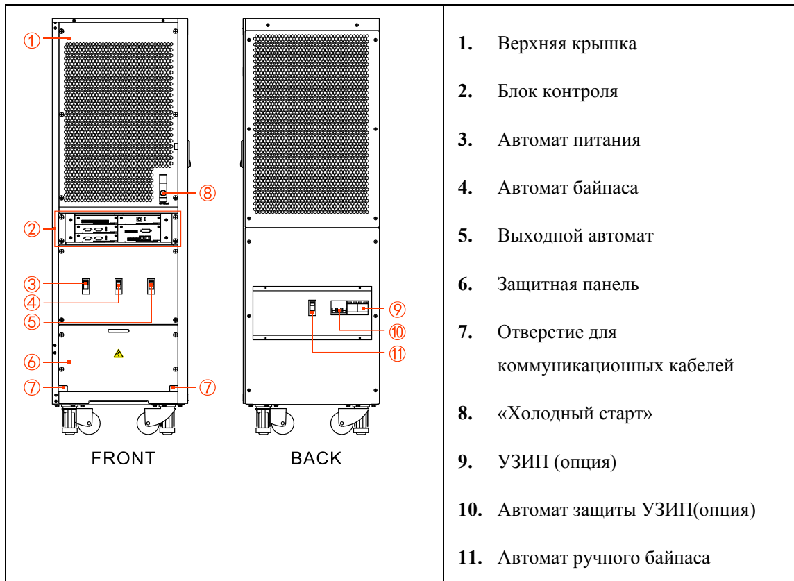
Рис 2.11 Структурная схема расположения для KR(/B)3380, KR(/B)33100, KR(/B)33120
