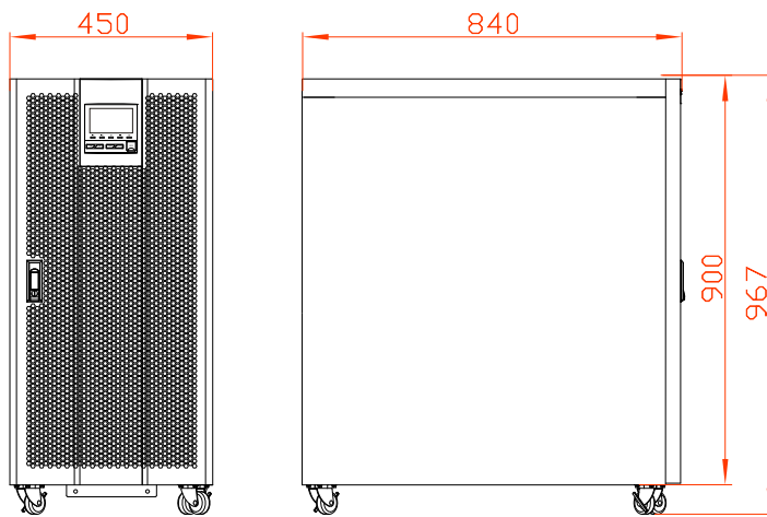
Рис 3.11 Размер для KR(/B)3350, KR(/B)3360
