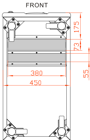
Рис 3.20 Схема нижних монтажных отверстий для KR(/B)3380, KR(/B)33100, KR(/B)33120
