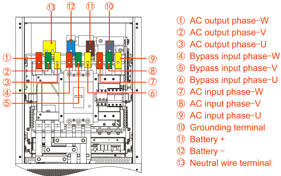
Рис 3.26 Схема подключения клемм для KR(B)33160, KR(B)33200 (back view)
