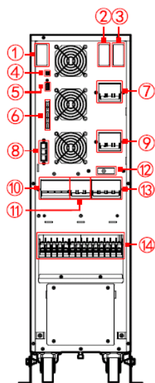
Рис 2-5 Вид задней панели моделей 10/10S/15/15S/20/20S
