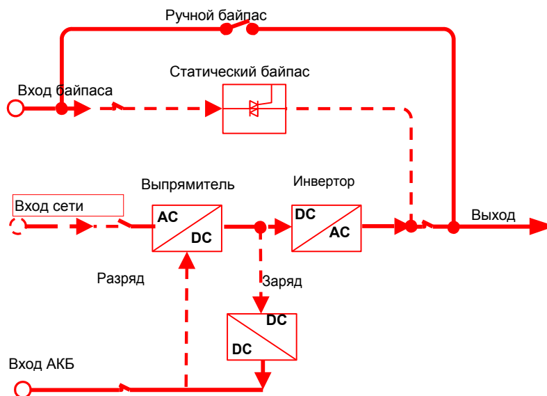
Рис 2-13 Режим ручного байпаса (жирная линия показывает поток энергии)
