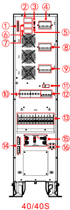
Рис 2-7 Вид задней панели моделей 40/40S
