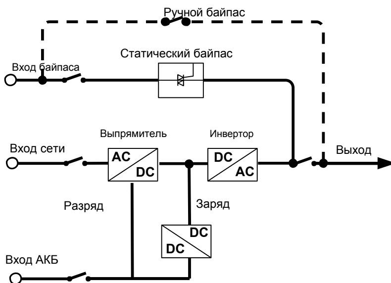
Рис. 2-9 Функциональная диаграмма
