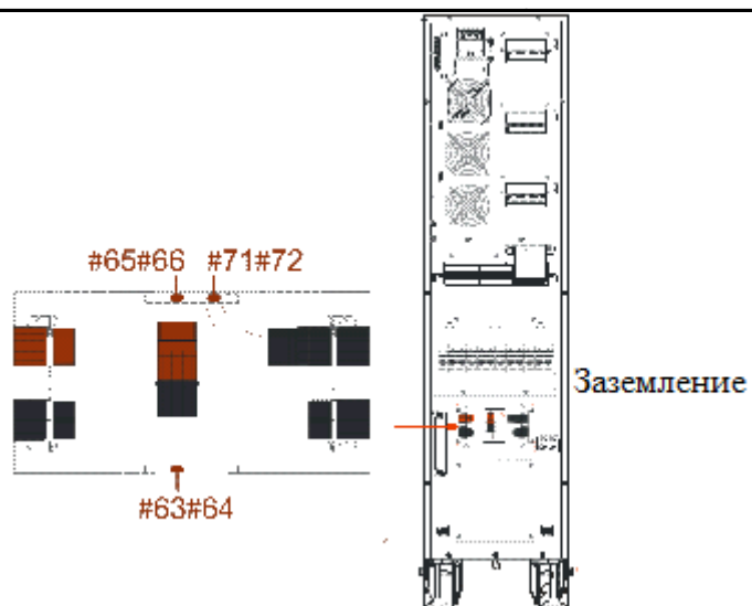
Рис. 3-20 Подключение установочной перемычки по умолчанию
