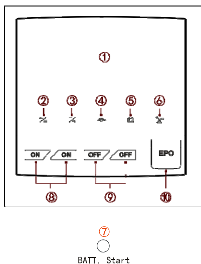
Рис 2-4 Панель управления с сенсорным дисплеем
