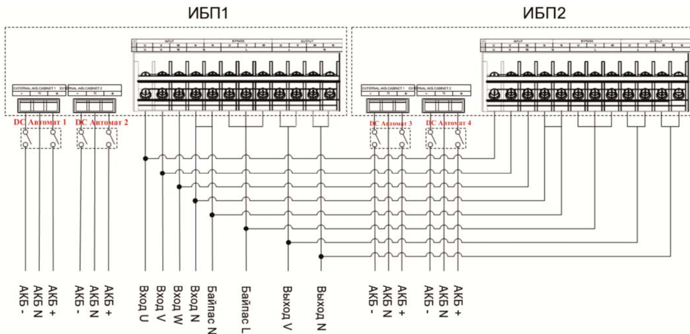
Рис. 3-30 30/30S/40/40S диаграмма подключения для 31 режима параллельной системы
