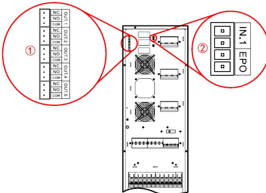
Рис 2-15 Расположение сухих контактов для ИБП 30/30S/40/40S
