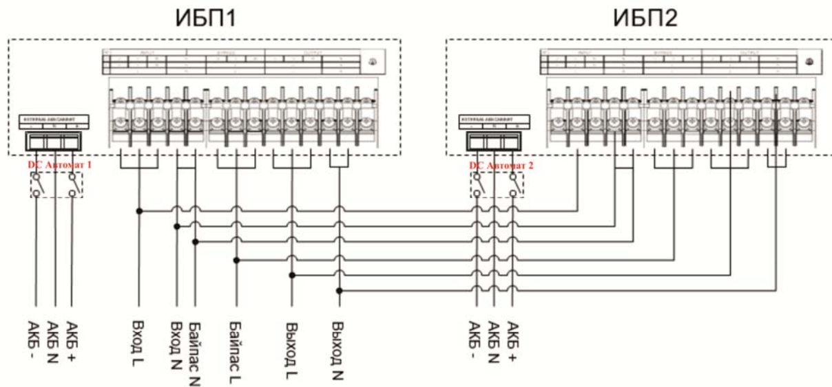
Рис. 3-28 10/10S/15/15S/20/20S диаграмма подключения для 11 режима параллельной системы
