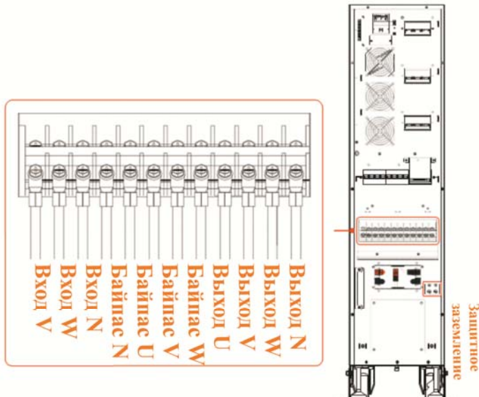
Рис. 3-21 Диаграмма подключения для 33 режима
