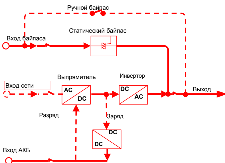
Рис 2-12 Режим работы через байпас ((жирная линия показывает поток энергии))
