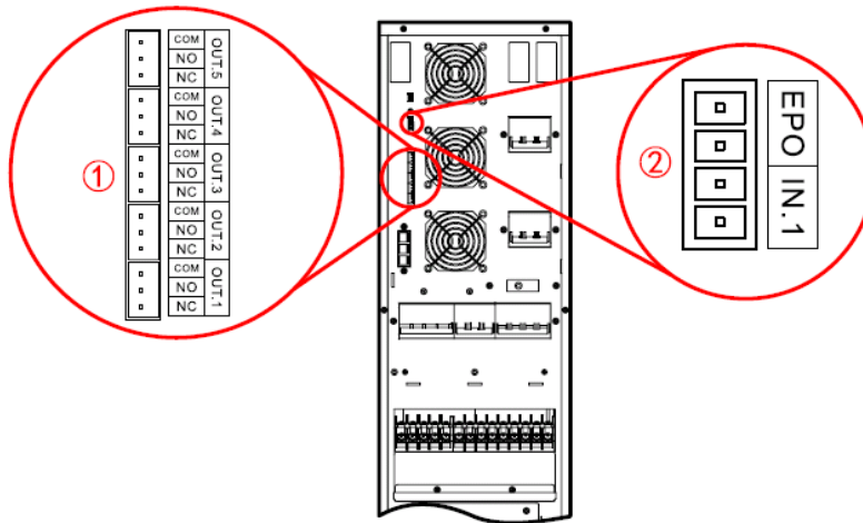
Рис 2-14 Расположение сухих контактов для ИБП 10/10S/15/15S/20/20S
